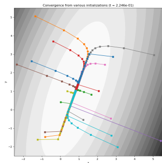
(d) Iterates for various preconditioners.
