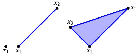
Abbildung 16.5.: Simples der Dimensionen 0, 1 und 2 im \mathbb{R}^2 .
