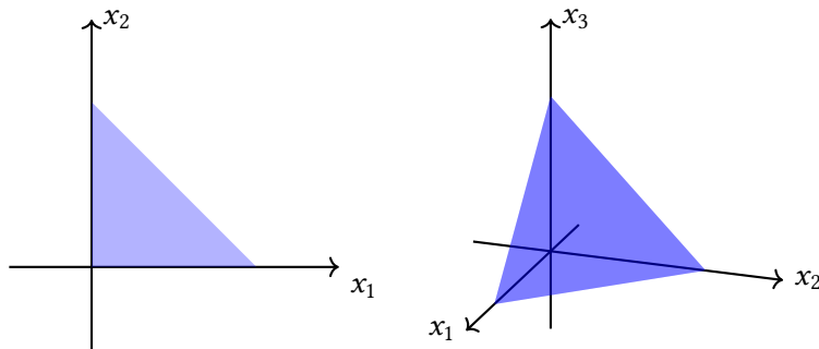
Abbildung 13.2.: Einheitsimplizes im \mathbb{R}^2 und \mathbb{R}^3 .
