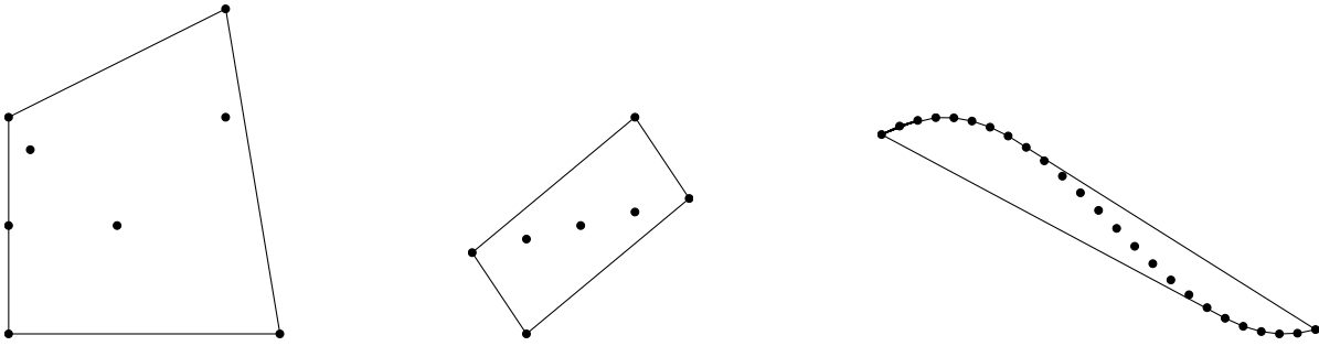
Abbildung 13.4.: Konvexe Hüllen einiger Punktmengeten in \mathbb{R}^2 .
